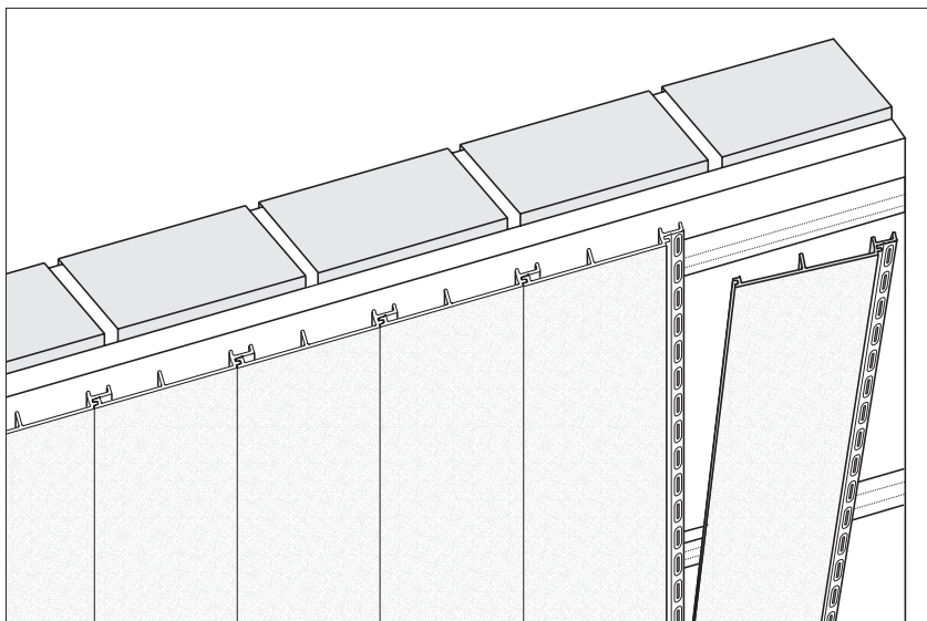
vinylTherm Fassadenprofile
